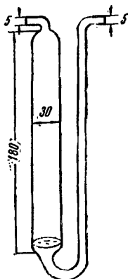
Рис. 1. Поглотительный прибор с пористой пластинкой.
