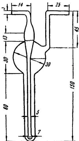
Рис. 7. Поглотительный прибор Полежаева.
