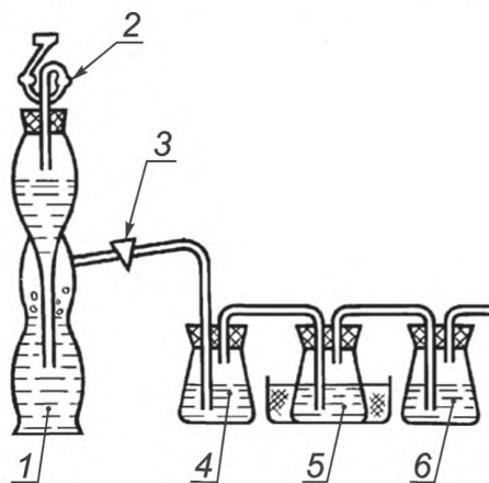
1 – аппарат Киппа; 2 – предохранительная воронка; 3 – кран; 4, 6 – промывная склянка; 5 – поглотительная склянка
