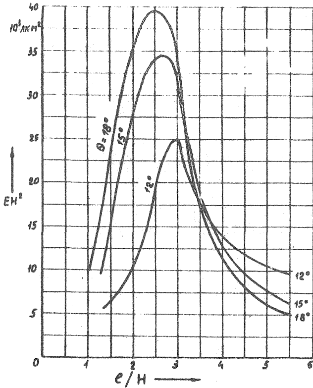
Рис. П.13.2. График для определения освещенности от группы прожекторов ПСМ-40-1 с лампой 500 Вт, 220 В (для \hat{c} = 1^\circ )
