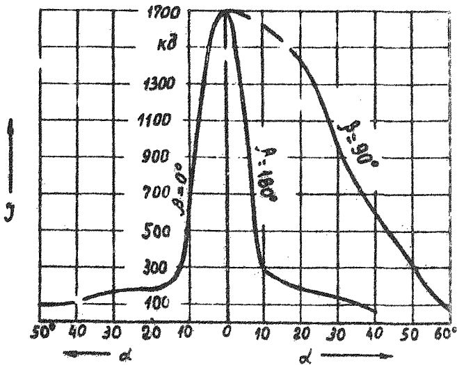
Рис. П.2.6. Кривые силы света светильника ИСУО2-5000
