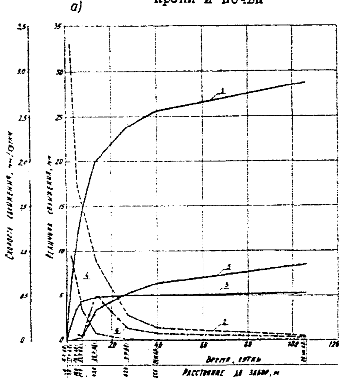
Рис. 5. Графики сближения пород контура и крепи в главных откаточных нвершлагах горизонта -620 м на шахте № 18 "Капитальная": а - в крепких песчаниках; б - в трещиноватых аргиллитах; 1-величина сближения кровли и почвы; 2-скорость сближения кровли и почвы; 3-величина сближения стенок; 4-скорость сближения стенок; 5-величина сближения свода крепи и почвы; 6-скорость сближения свода крепи и почвы
