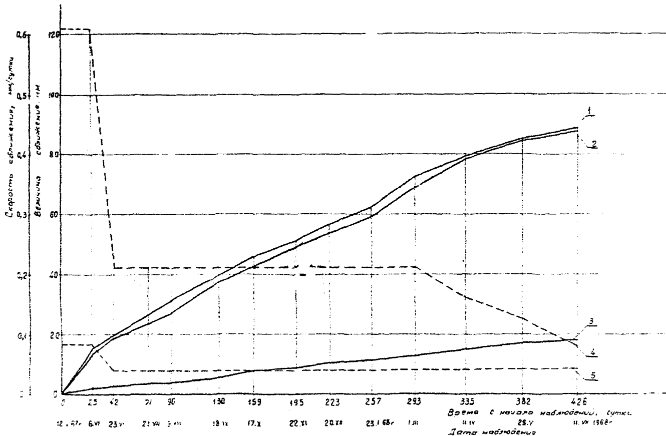
рис. 12. Графики сближения реперов в южном полевом штреке на шахте № 40: 1—сближения кровли и почвы со стороны падения пласта; 2—сближения кровли и почвы со стороны восстания; 3—сближения стенок выработки; 4—скорость сближения кровли и почвы со стороны падения; 5—скорость сближения стенок выработки
