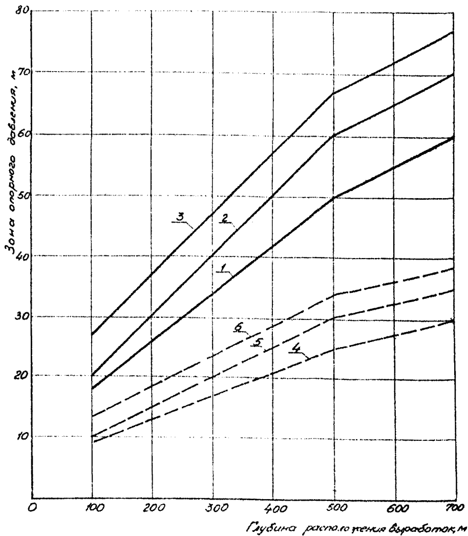
Рис. 2. Графики зон опорного давления и интенсивного смещения. Зоны опорного давления при мощности пласта: 1—до 1,7 м; 2—от 1,7 до 2,9 м; 3—более 2,9 м. Зоны интенсивного смещения при мощности пласта: 4—до 1,7 м; 5—от 1,7 до 2,9 м; 6—более 2,9 м
