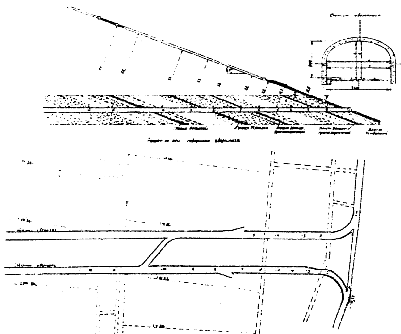
Рис. 8. Схема заложения наблюдательной станции в северном отка- точном квершлагае горизонта - 510 м на шахте № 40; 1-12-номера реперов
