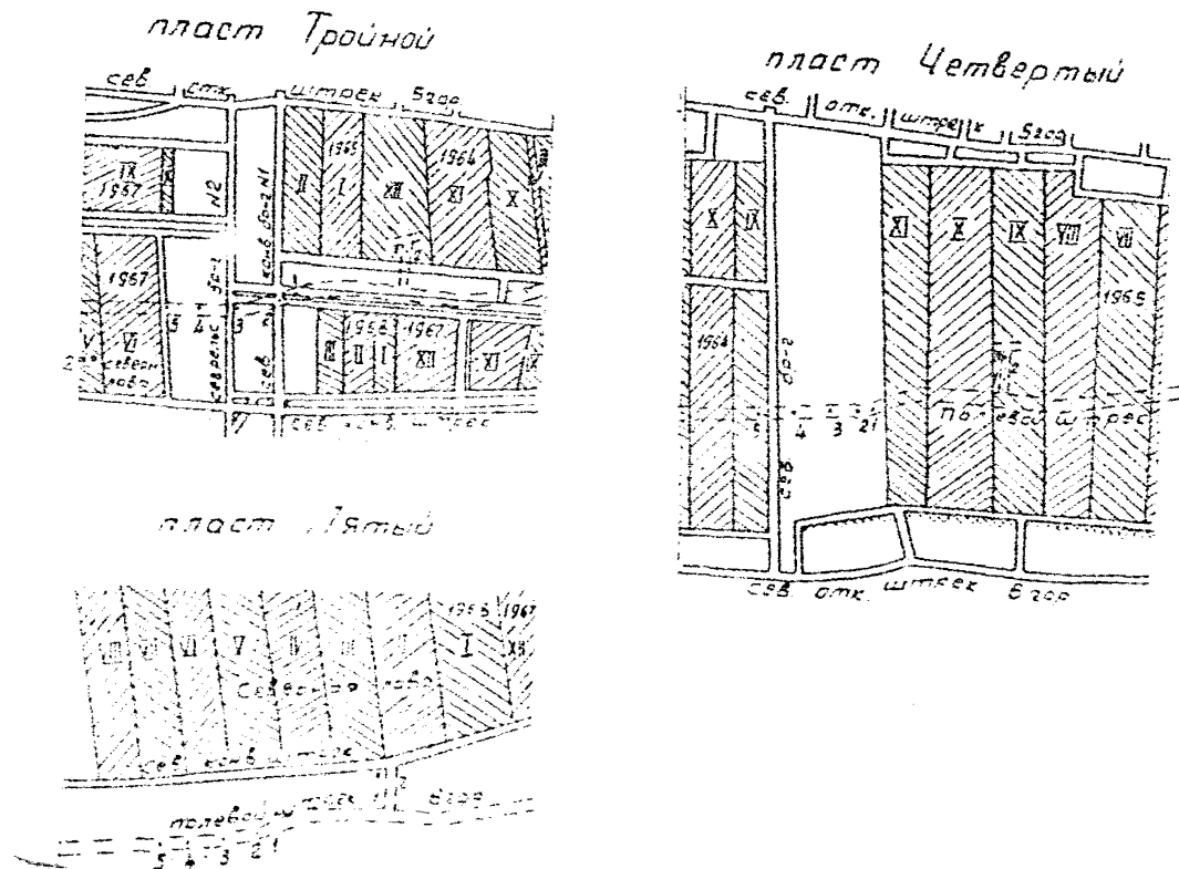
Рис. 13. Схема заложения наблюдательных станций в северном поле штреке на шахта № 5. 1-5 - номера реперов
