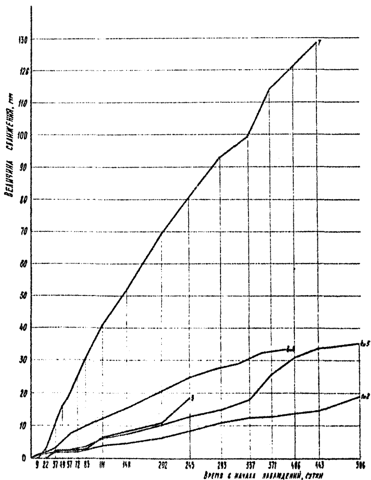
Рис. II. Графики сближения реперов кровли и почвы южного полевого дренажа на шахте № I "Капитальная": 1-8-номера реперов
