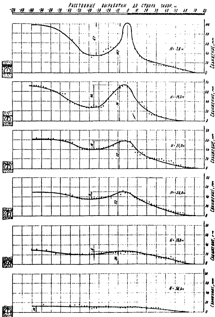
Рис. 18. Графики величин сближения кровли и почвы выработок при надработке пластом Четвертым: 1-7-номера выработок 43
