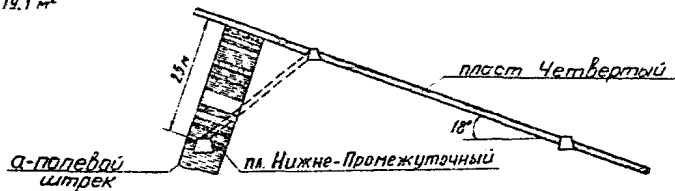
Рис. 10. Схема заложения наблюдательной станции в южном полевом штреке на шахте № I "Капитальная"
