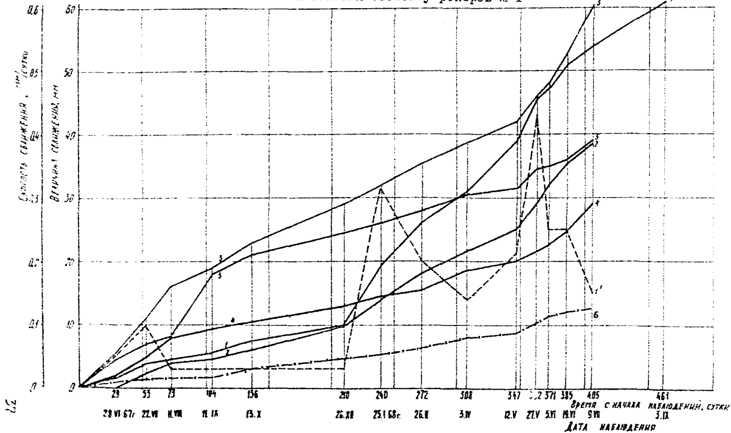
Рис. 14. Графики сближения реперов в северном полевом штреке на шахте № 5: 1-5 - величины сближения кровли и почвы; 1' - скорость сближения реперов № 1; 6 - величина сближения боковых стен у реперов № 1
