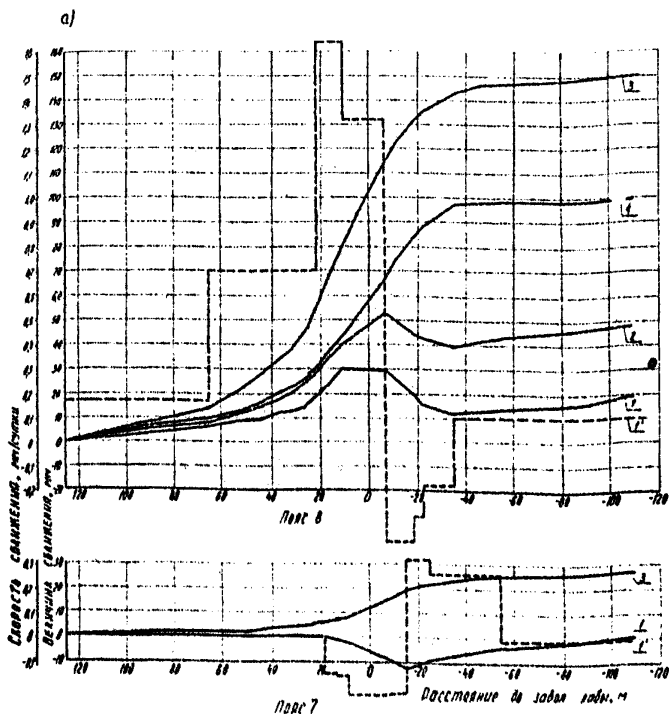
Рис. 9. Графики величин и интенсивности смещения пород контюра и крепи северного квершлага гор. - 510 м на шахте № 40
