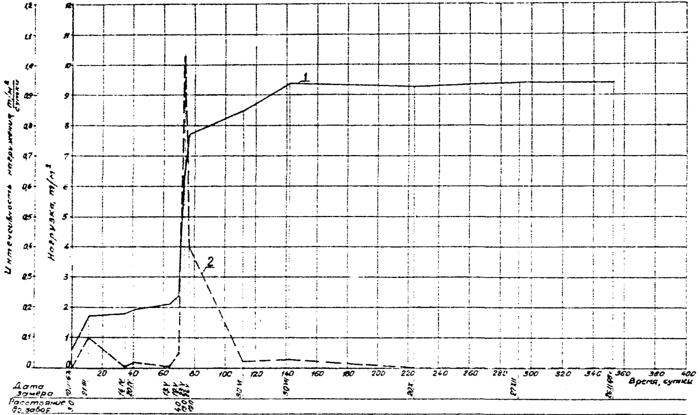
Рис. 7. Графики величин и интенсивности нагрузки на свод крепи посадочной площадки клетьевого ствола горизонта -620 м на шахте № 18 "Капитальная": 1—величина нагрузки; 2—интенсивность нагрузки
