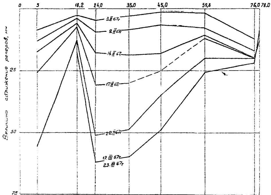
Рис. 16. Графики величины сближения кровли и почвы по квершлагу № 9 на шахте № I "Капитальная"
