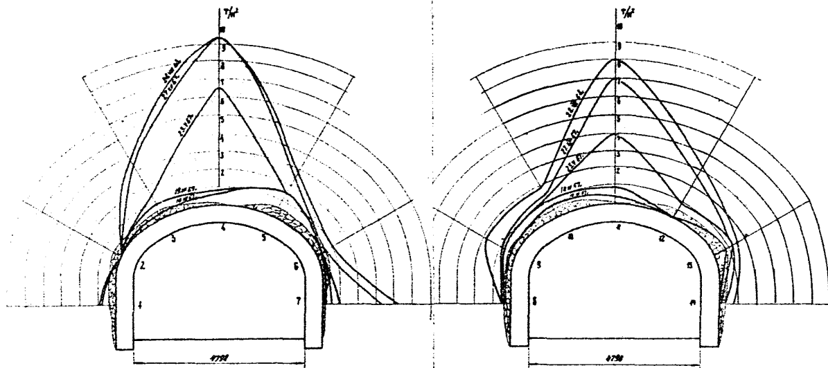
Рис. 6. Эпюры нагрузки на крепь посадочной площадки клетового ствола горизонта - 620 м на махте № 18 "Капитальная": I-I4 -номера динамометров
