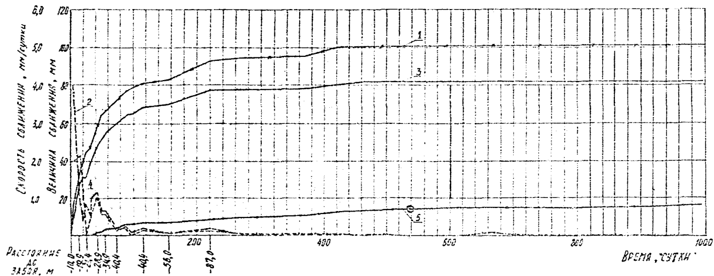
Рис. 4. Графики сближения пород контура и крепи в северной обгонной выработке околоствольного двора горизонта - 620 м на шахте № 18 "Капитальная": 1-величина сближения кровли и почвы; 2-скорость сближения кровли и почвы; 3-величина сближения свода крепи и почвы; 4 - скорость сближения свода крепи и почвы; 5 - величина сближения стенок крепи на уровне 0,7 м от почвы
