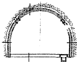
Сечение по I-I
