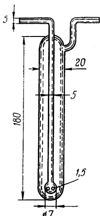
Рис. 1. Поглощительный прибор Петри
