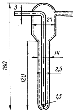
Рис. 2. Поглощительный прибор Зайцева
