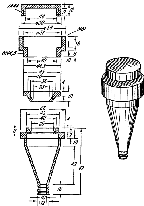
Рис. 12. Металлический патрон для бумажного и других фильтров.
