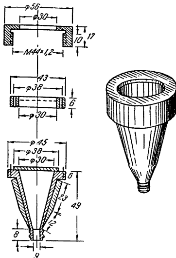
Рис. 13. Плексигласовый патрон для бумажного и других фильтров.
