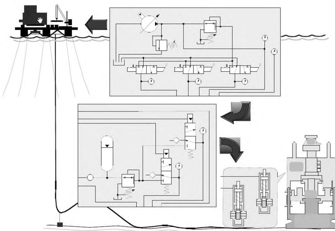
Рис. 3 Гидравлические системы с подводным управляющим модулем
