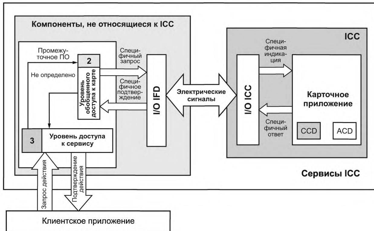
Рисунок А.3 — Объединенная реализация
