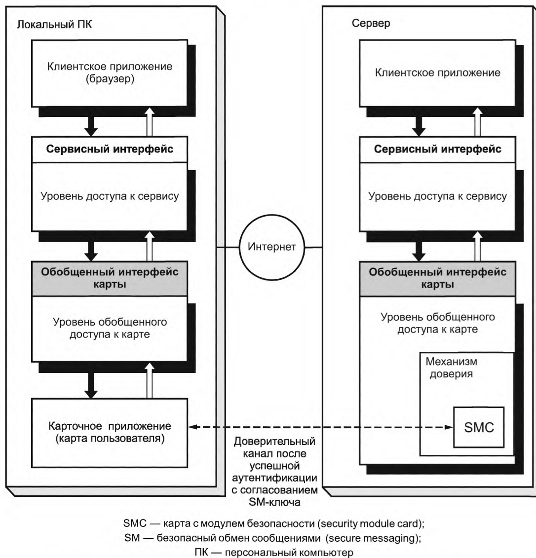
Рисунок А.10 — Распределенная реализация, использующая механизм доверия
