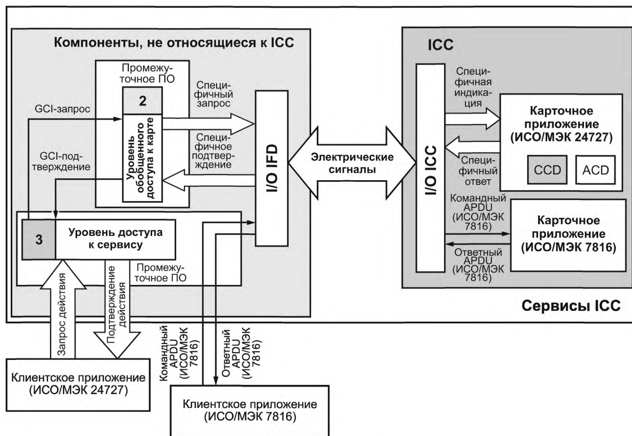
Рисунок А.8 — Конфигурация со множеством приложений
