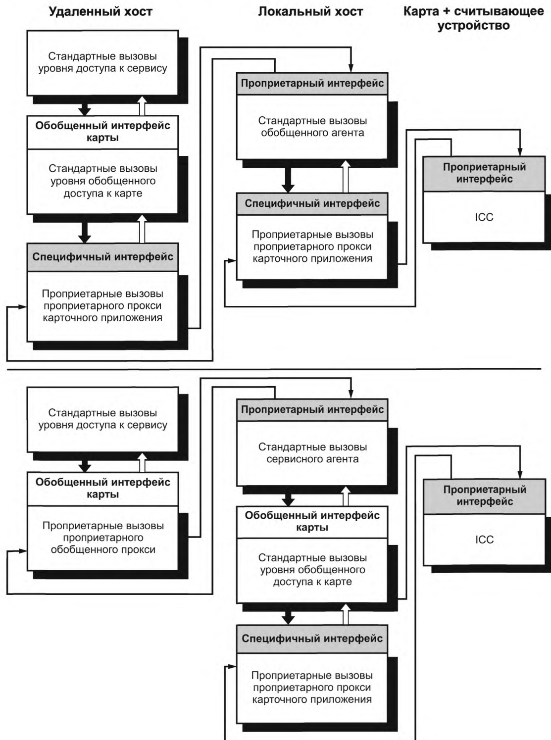
Рисунок А.9 — Распределенная реализация стека
