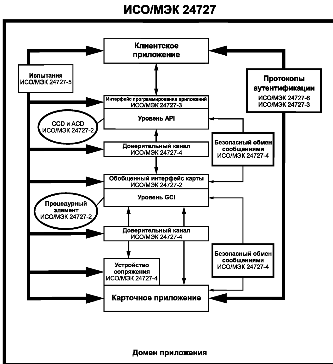
Рисунок 1 — Логическая архитектура по стандартам серии ИСО/МЭК 24727
