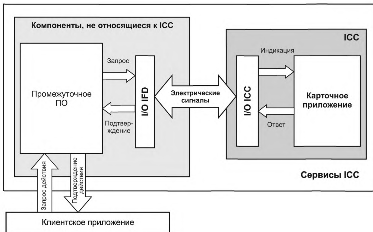
Рисунок А.1 — Физическая архитектура
