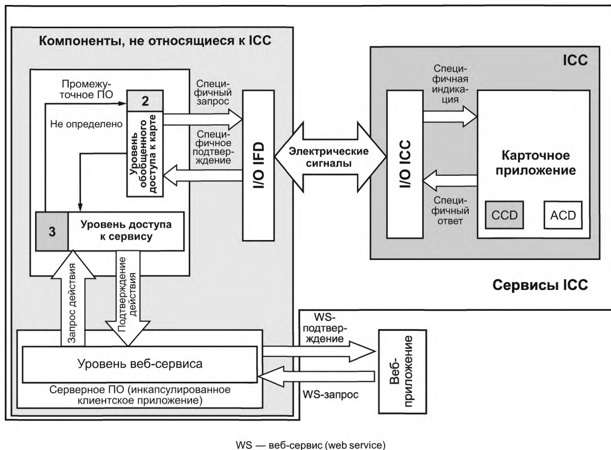
Рисунок А.7 — Конфигурация с использованием веб-сервиса
