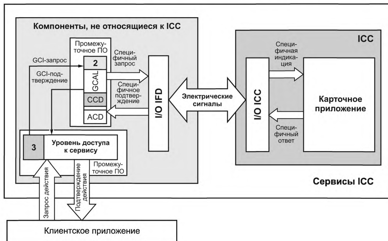
Рисунок А.6 — Загружаемая или фиксированная конфигурация
