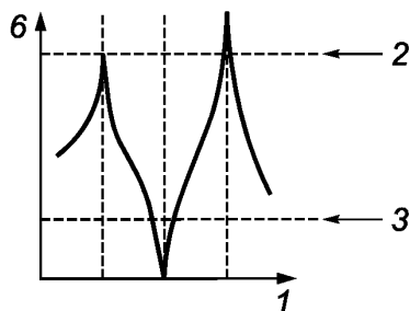
в) Возбуждение с постоянной амплитудой
