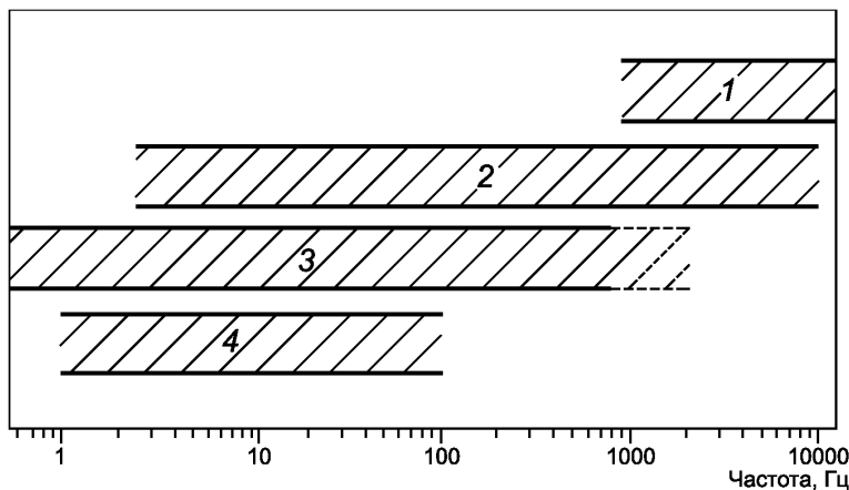
1 — пьезоэлектрические; 2 — электродинамические; 3 — гидравлические; 4 — механические
