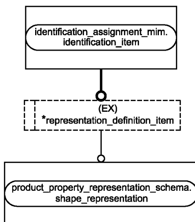
Рисунок D.2 — Представление ИММ на уровне объектов в формате EXPRESS-G
