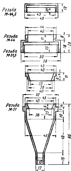
Рис. 1. Металлический патрон.
