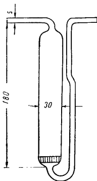
Рис. 5. Поглощительный прибор с пористой пластинкой.
