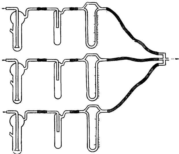
Рис. 7. Схема отбора проб воздуха на ЦТМ.
