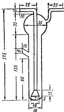
Рис. 6. Поглощительный прибор Яворовской.
