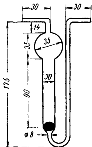
Рис. 8. Погло- тельный прибор с пористой пластин- кой.
