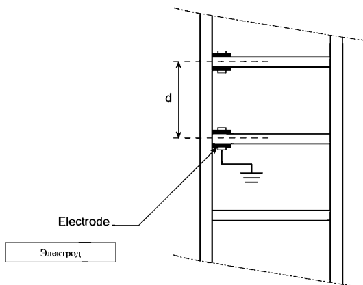
Рис. 9. Схема электрических испытаний.
