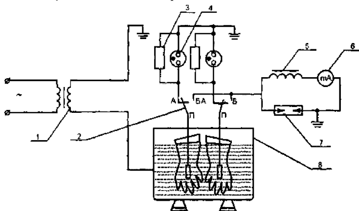
Рис. 11. Принципиальная схема испытания диэлектрических перчаток:
