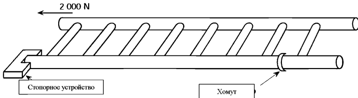
Рис. 8. Испытания перекладин/тетив в сборе.
