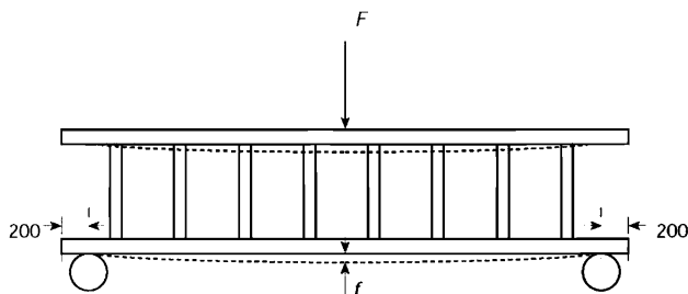
Рис. 5. Испытания на боковой прогиб.
