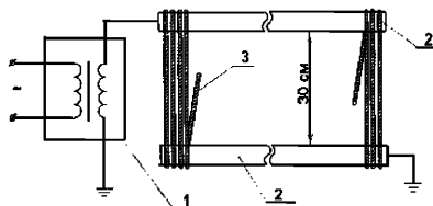
Рис. 3. Схема электрических испытаний изолирующего каната:
