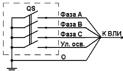
Рис. 13. Схема стационарного устройства заземления
