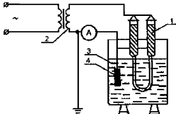
Рис. 1. Принципиальная схема испытания электрической прочности изоляции рукояток и провода указателя напряжения:
