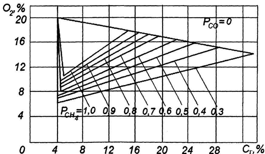
Рис. 1. Треугольник взрываемости при P_{CO} = 0,0
