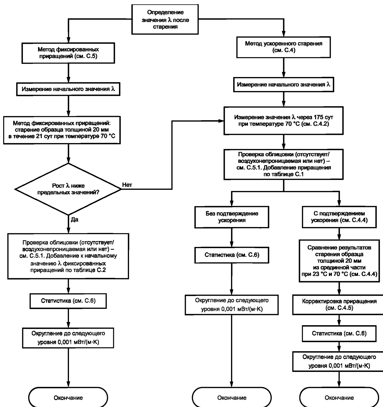
Рисунок С.1— Блок-схема альтернативных методов старения
