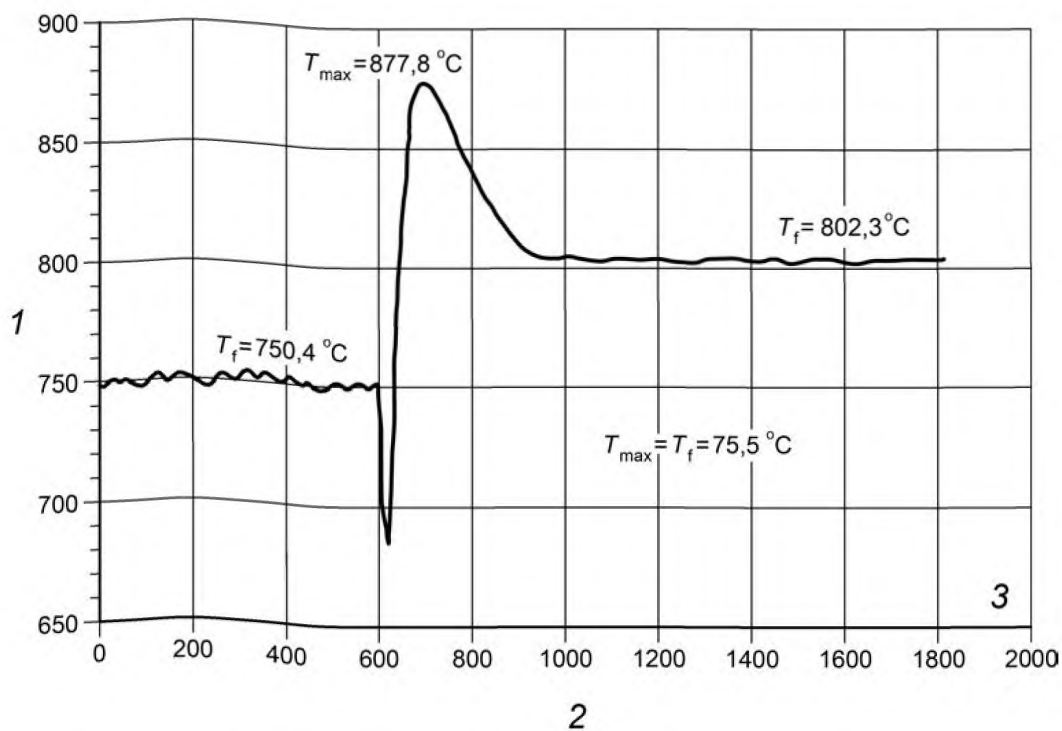
Рисунок Б.3 — Пример записи температуры во время испытания А
