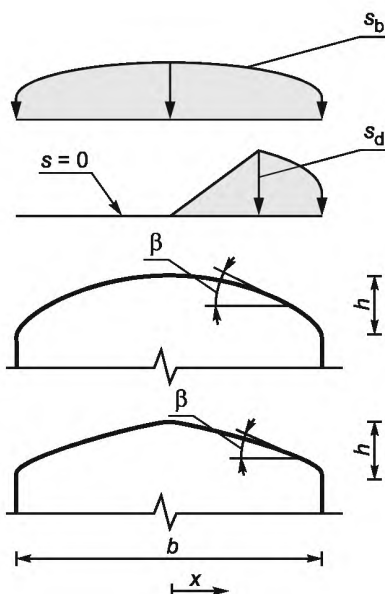
Рисунок В.5 — Распределение базовой нагрузки и нагрузки от переноса для криволинейных покрытий
