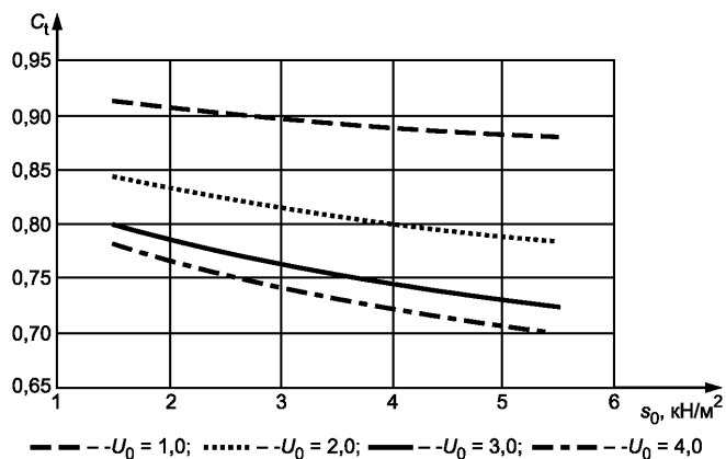
Рисунок D.1 — Термический коэффициент C_t при \theta = 10\text{ }^{\circ}\text{C}
