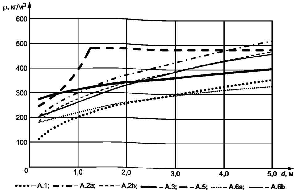
Рисунок А.1 — Плотность снега \rho как функция высоты снегового покрова d в формулах (А.1), (А.2), (А.3), (А.5) и (А.6)
