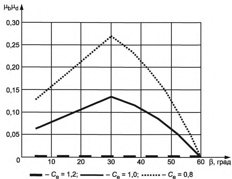
Рисунок В.2 — Произведение \mu_b \mu_d как функция уклона покрытия \beta при C_m = 1,0
