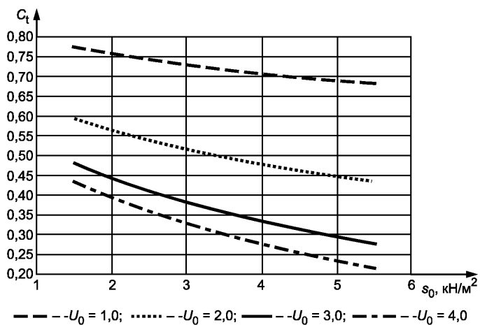
Рисунок D.3 — Термический коэффициент C_t при \theta = 18\text{ }^{\circ}\text{C}
