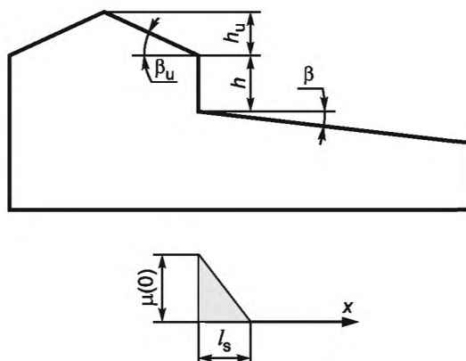
Рисунок В.12 — Коэффициент сползания снеговой нагрузки
