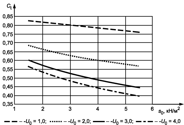
Рисунок D.2 — Термический коэффициент C_t при \theta = 15\text{ }^{\circ}\text{C}
