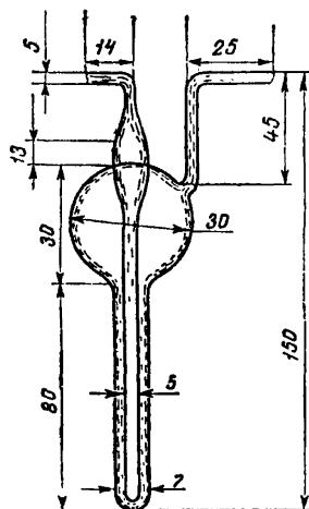
Рис. 8. Поглощительный прибор Полежаева
