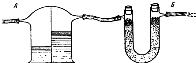
Рис. 13. Очистительная система а — склянка Тищенко с серной кислотой; б — поглотитель с натронной известью
