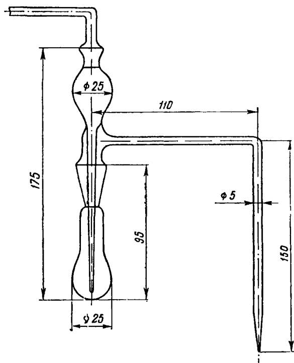
Рис. 12. Прибор для сжигания хлорорганических ядохимикатов
