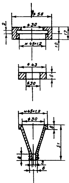
Рис. 2. Плексигласовый патрон для фильтра
