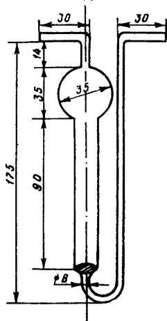
Рис. 3. Поглотительный прибор с пористой пластинкой
