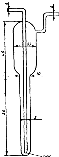
Рис. 5. Поглотительный прибор Зайцева (малый)
