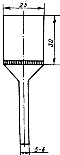
Рис. 7. Воронка стеклянная с пористой пластинкой
