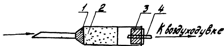
Рисунок. Схема концентрационной трубки: 1 - стеклянная вата; 2 - окись алюминия; 3 - резиновая пробка; 4 - стеклянная трубка
