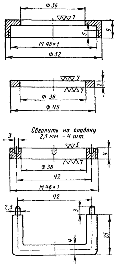
Рис. 3. Металлическая кассета для закрепления фильтров
