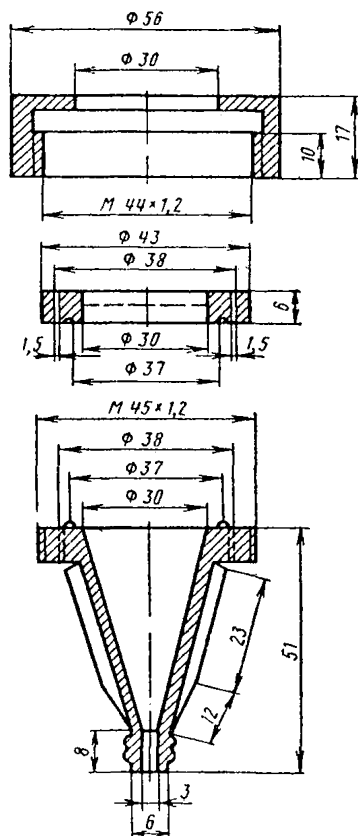
Рис. 4. Плексигласовый патрон для фильтров
