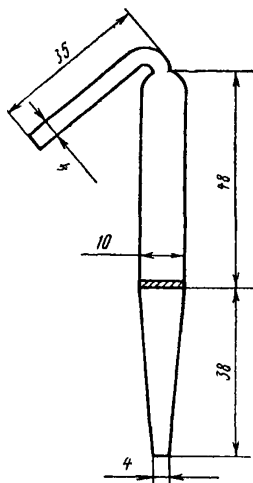
Рис. 5. Стеклообразующая трубка с пористой пластинкой для отбора проб воздуха
