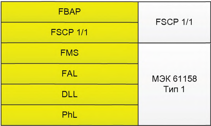
Рисунок 11 — Связь между FSCP 1/1 и другими уровнями МЭК 61158, Тип 1
