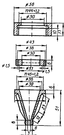
Рис. 7. Плексигласовый патрон
