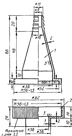
Рис. 4. Металлический патрон Рис. 5. Металлический патрон, употребляемый с кассетой
