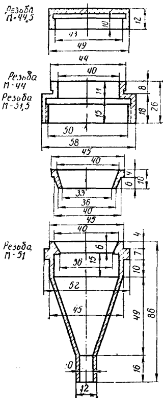
Рис. 4. Металлический патрон Рис. 5. Металлический патрон, употребляемый с кассетой
