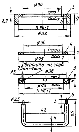
Рис. 6. Металлическая кассета для закрепления фильтров
