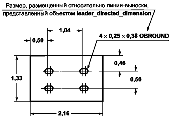
Рисунок 8 — Размер, размещаемый относительно линии-выноски
