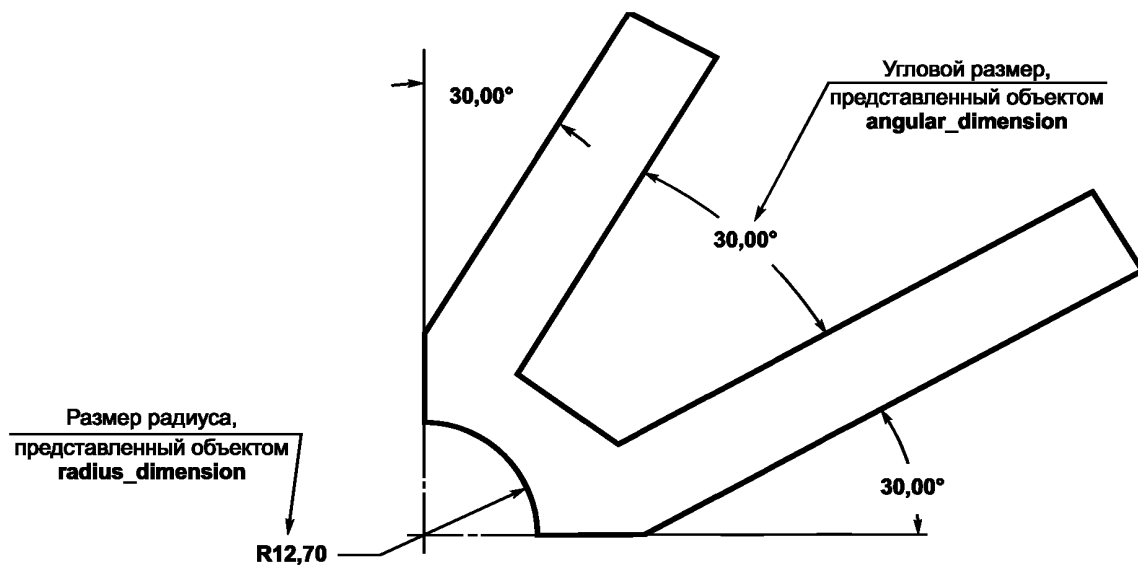
Рисунок 1 – Угловые размеры и размер радиуса
