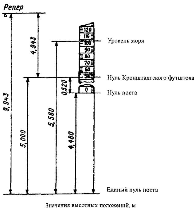
Рисунок 1 – Пример высотных положений условных поверхностей
