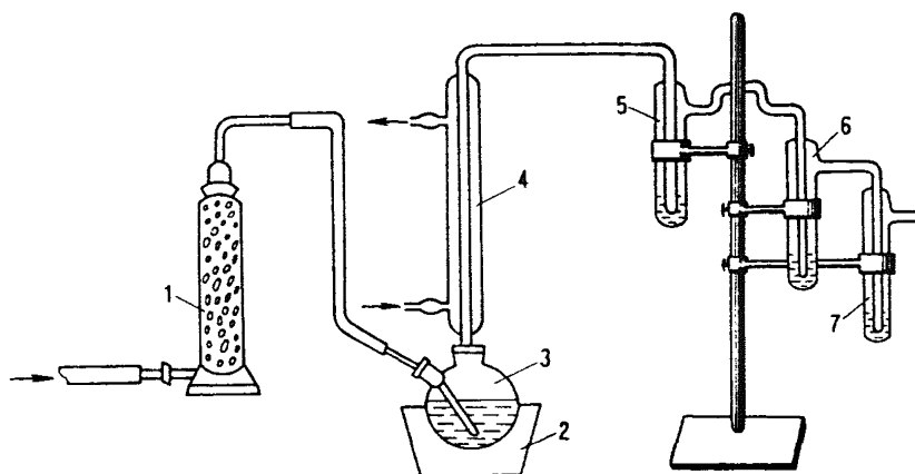
Рис. 9. Прибор для выделения сероуглерода из цинсба:
