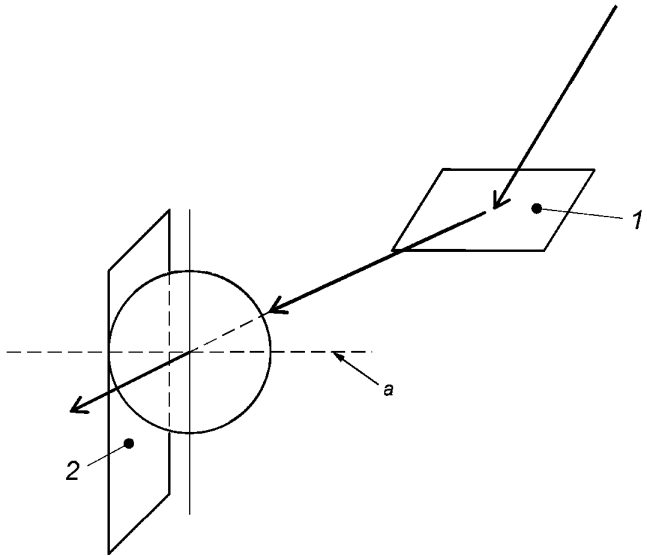
1 — горизонтальная отражающая поверхность; 2 — вертикальная плоскость пропускания светофильтра;
