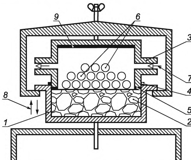
1 — испытательная камера; 2 — испытуемый образец; 3 — крышка испытательной камеры; 4 — круглая кольцообразная резиновая прокладка; 5 — плоская кольцообразная резиновая прокладка; 6 — стальные шары; 7 — движение воды; 8 — направление хода поршня; 9 — круглая резиновая пластина
