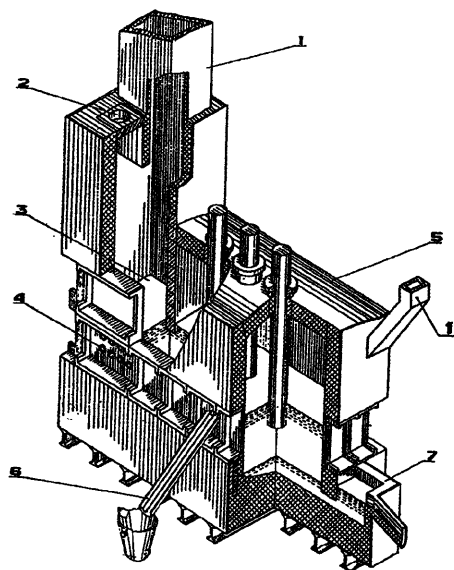
1 — стояк; 2 — загрузка; 3 — плавильная шахта; 4 — фурмы; 5 — электроотстойник; 6 — выпуск шлака; 7 — сифонный выпуск свинца
