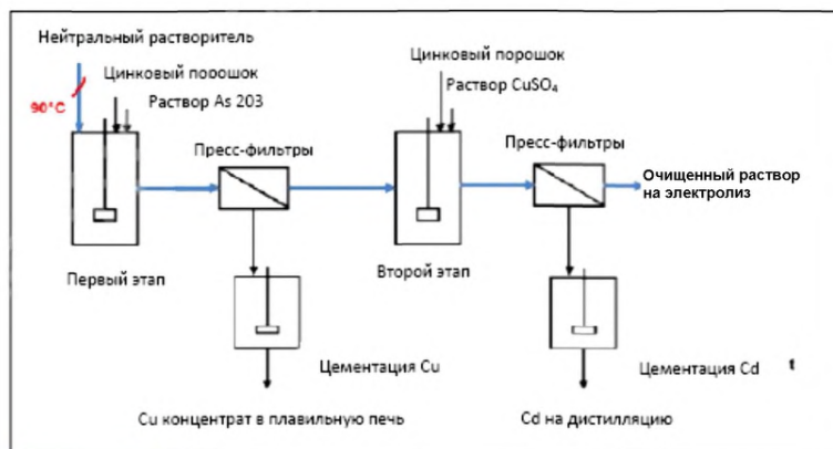
Рисунок 2.14 — Пример схемы процесса очистки, основанного на \text{As} , для удаления \text{Co} и \text{Ni}
