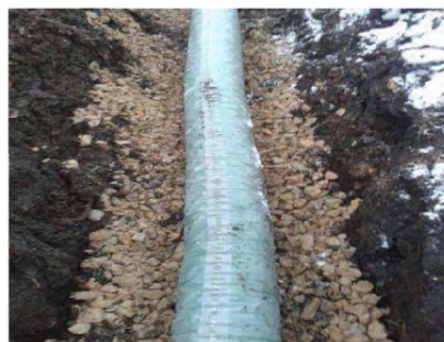
Рис. 2.12 — Газосборная траншея с дренажной трубой (Пермский край) ([47])
