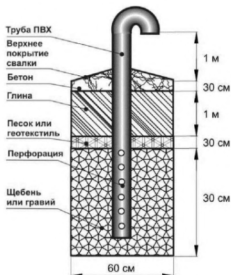
Рис. 2.13 — Газовыпуск при устройстве траншейной системы сбора биогаза ([46])
