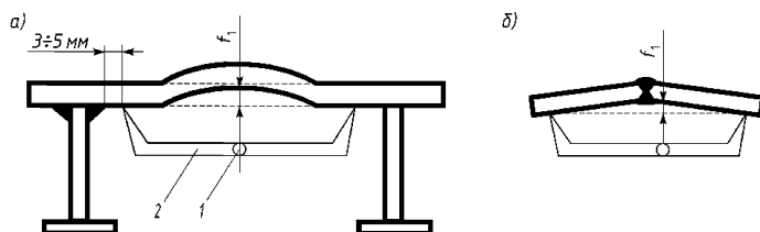
Рис. 3.1.27. Измерение отклонений цилиндрических и конических оболочек от правильной формы: a — по образующей между шпангоутами;
