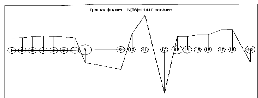
Рис. ПЗ.3-12. График амплитуд свободных колебаний 6-узловой формы
