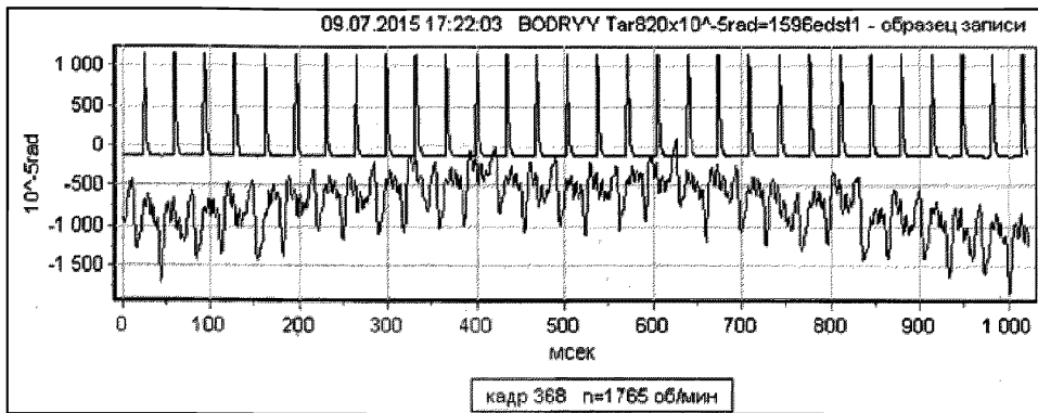
Рис. П3.2-9 Образец 6 записи торсионграммы
