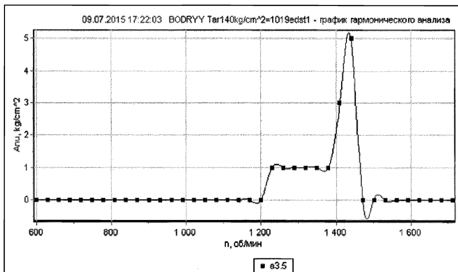
Рис. ПЗ.2-13 График 3 гармонического анализа при работе на FiFi с максимальной нагрузкой. Усредненные амплитуды колебаний
