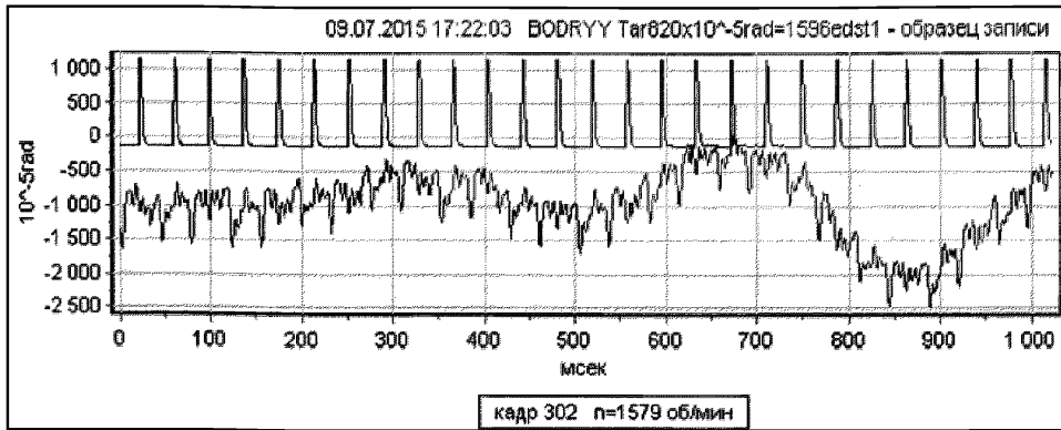
Рис. П3.2-8 Образец 5 записи торсионграммы
