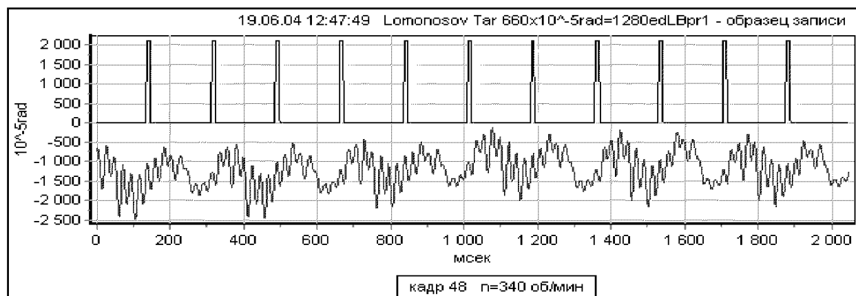
Рис. П2.2-5. Образец 2 записи торсионной диаграммы
