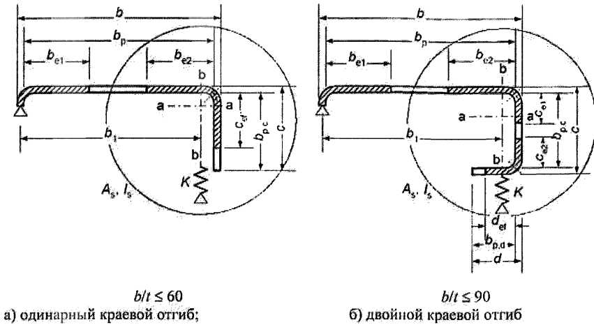
Рисунок 7.8 – Краевые отгибы
