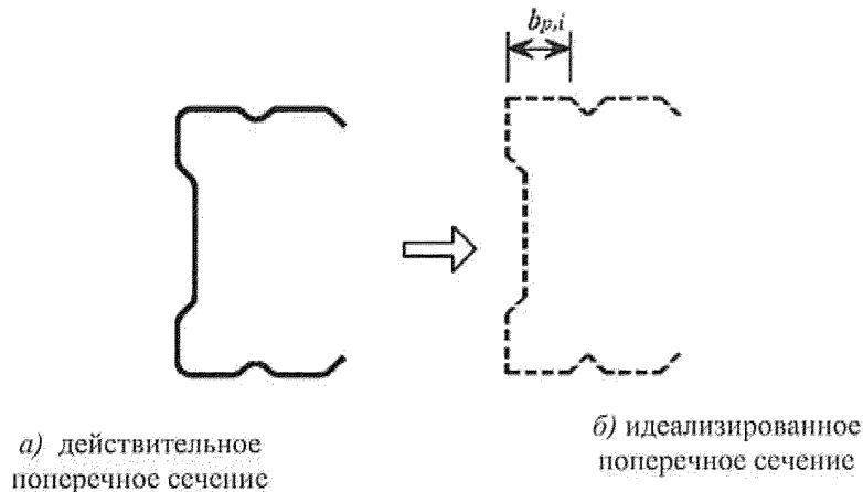
Рисунок 7.4 – Приближенные допущения для углов сгиба
