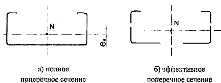
Рисунок 7.15 – Эффективное поперечное сечение при сжатии
