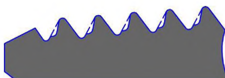
а) Подрез боковой стороны витка
