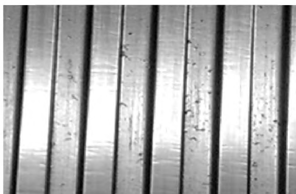
б) Раковина, образовавшаяся на наружной резьбе после выпадения крупного неметаллического включения
