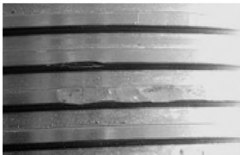
а) Вмятина на вершине витка наружной резьбы
