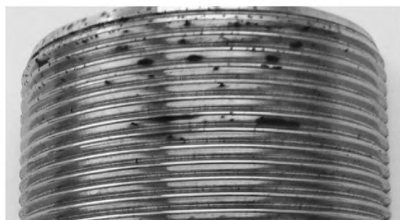
б) Следы коррозии на наружной резьбе
