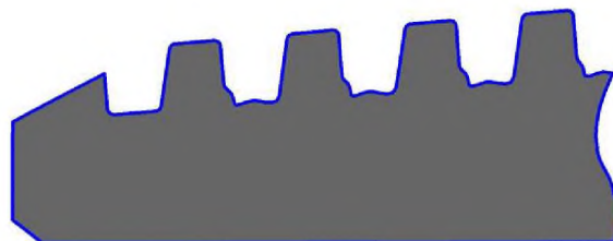
б) Уступы во впадинах витков трапецидальной резьбы
