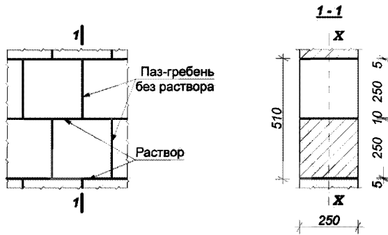
Рисунок Б.4.4 – Расчетное сечение кладки
