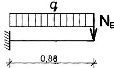
Рисунок Б.4.4 – Расчетная схема консоли схемы 1-1
