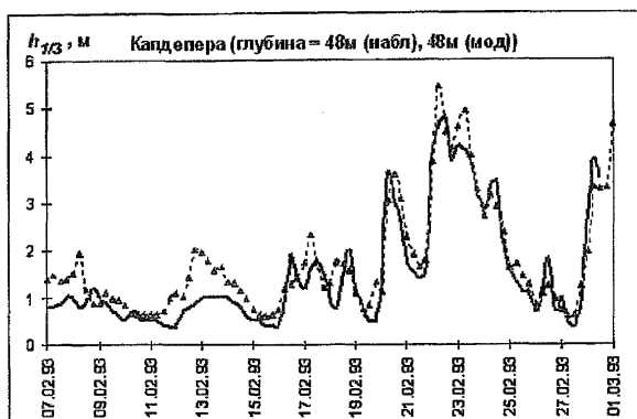
Рис. 6.6. Сопоставление измеренных и рассчитанных значительных высот волн в точках расположения буйев в Средиземном море.
