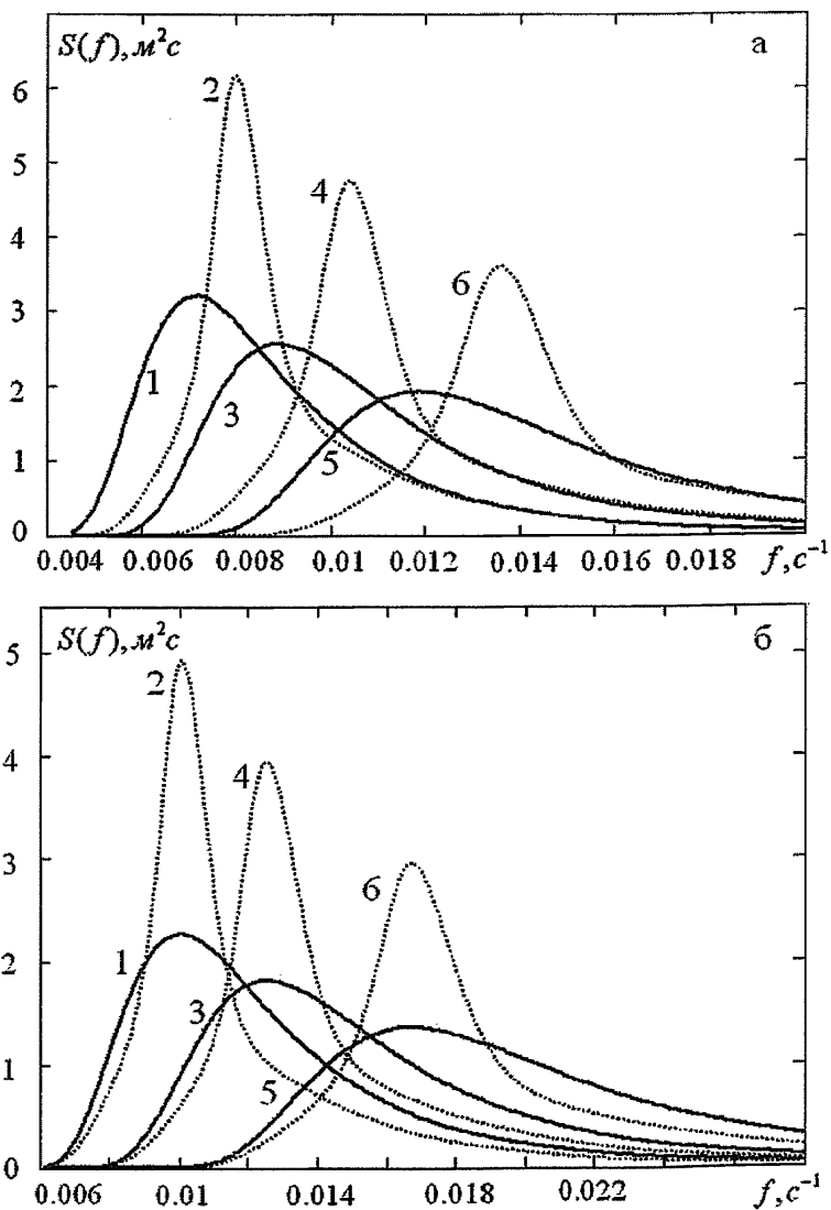
Рис. 3.1. Сопоставление частотных спектров Пирсона–Московица (ПМ) и JONSWAP. Высота волны h_{1/3} = 4 м. а) 1 - ПМ, 2 - JONSWAP T_z = 10c ; 3 - ПМ, 4 - JONSWAP T_z = 8c ; 5 - ПМ, 6 - JONSWAP T_z = 6c ; б) 1 - ПМ, 2 - JONSWAP T_p = 10c ; 3 - ПМ, 4 - JONSWAP T_p = 8c ; 5 - ПМ, 6 - JONSWAP T_p = 6c .
