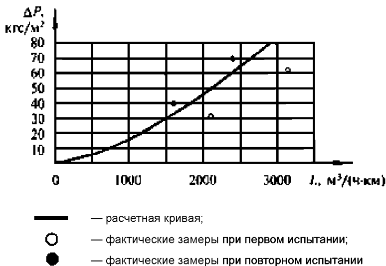
Рисунок В.3 — График характеристики герметичности отсека
