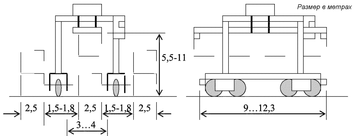
Рисунок 3 — Портальный автопогрузчик
