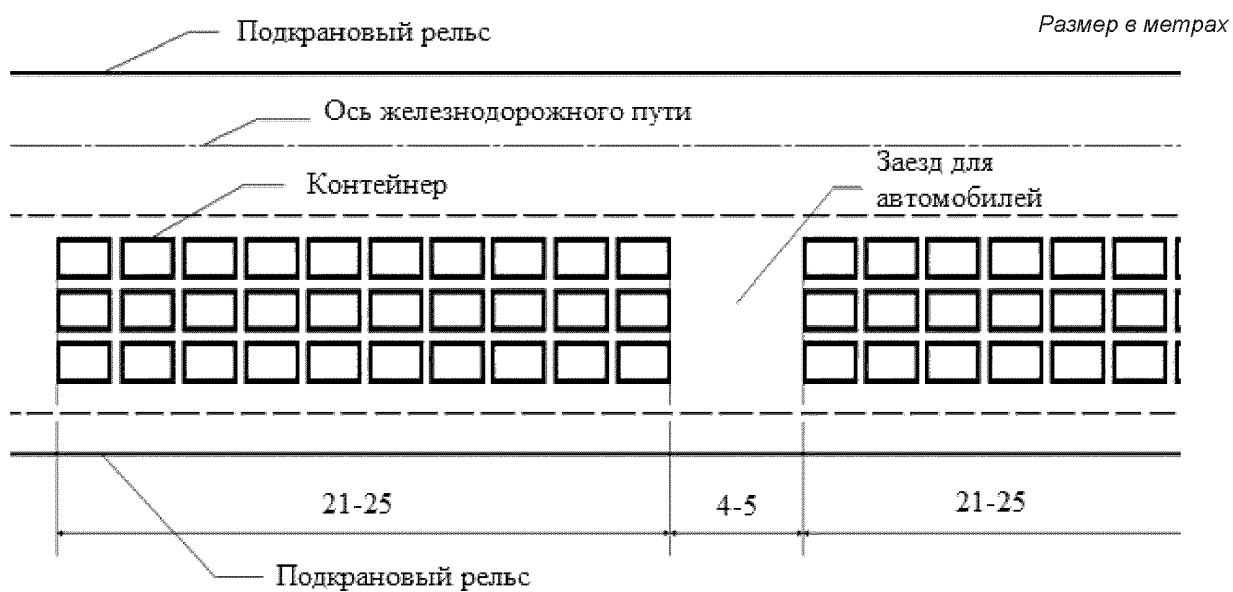
Рисунок 4 — Схема поперечного заезда автомобилей
