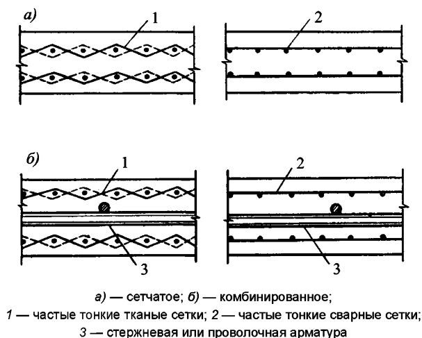
Рисунок 4.1 — Армирование армоцементных конструкций
