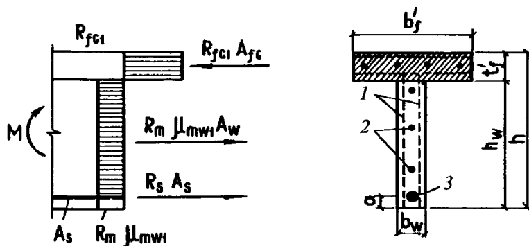
Рисунок 6.6 — Схема усилий и эпюра напряжений в изгибаемых элементах таврового сечения с полкой в сжатой зоне при x \leq t'_f
