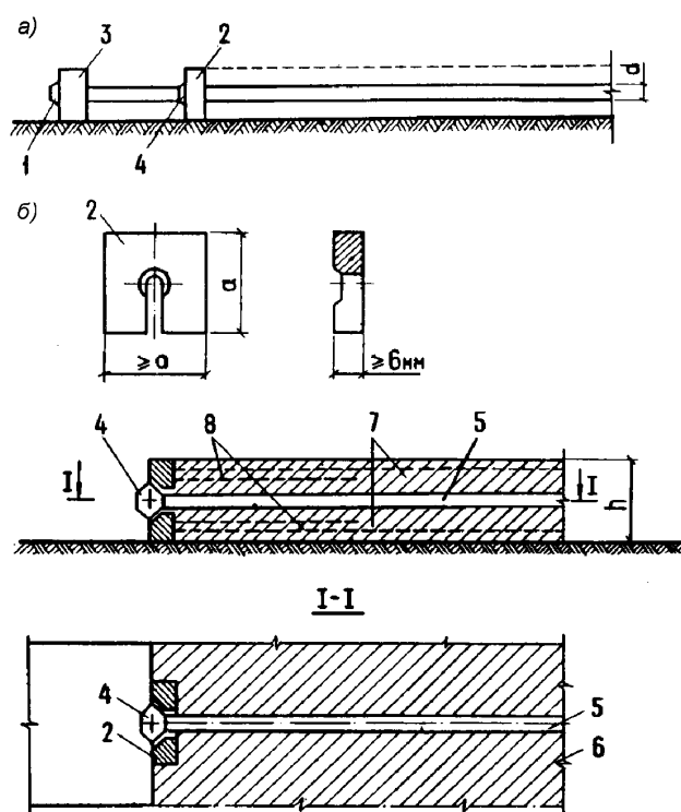
а) — напрягаемая арматура, заанкеренная на упорах формы; б) — элемент после отпуска предварительного напряжения арматуры; 1 — высаженная головка на конце проволоки; 2 — анкерная шайба с прорезью; 3 — неподвижный анкерный упор; 4 — промежуточная высаженная головка; 5 — проволока; 6 — предварительно напряженный элемент; 7 — основные сетки; 8 — дополнительные сетки
