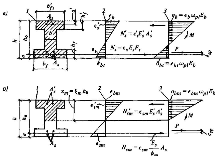
а) — участки, где в растянутой зоне отсутствуют трещины, нормальные к продольной оси; б) — участки, где в растянутой зоне имеются трещины, нормальные к продольной оси; 1 — сечения; 2 — эпюры деформаций; 3 — схемы усилий и эпюры напряжений
