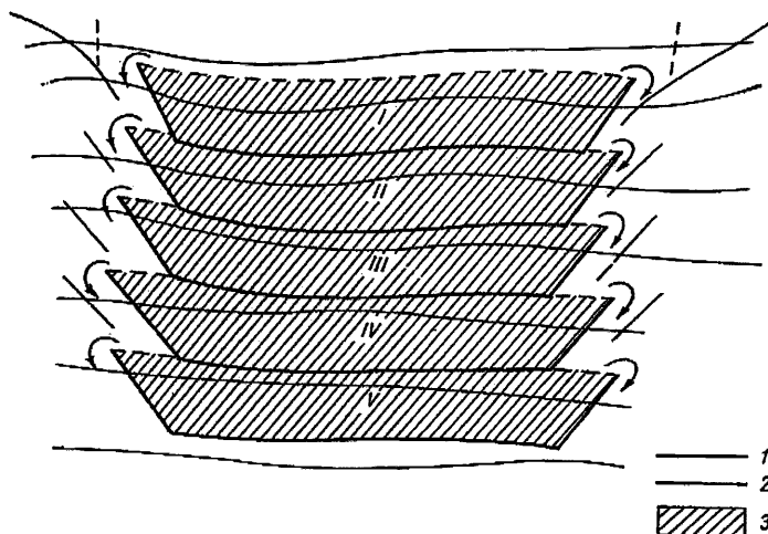
Рисунок Л.1 – Система лиманов на водораздельном плато
