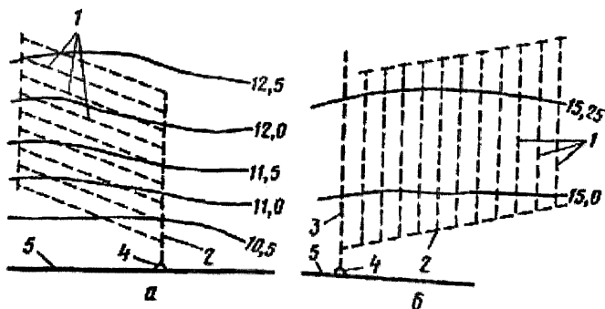
Рисунок III.1 – Схемы расположения закрытой регулирующей сети в плане
