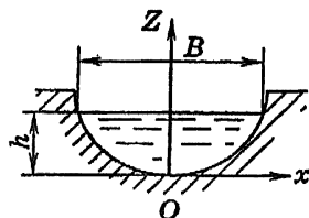
Рисунок Н.3 – Схема канала параболической формы
