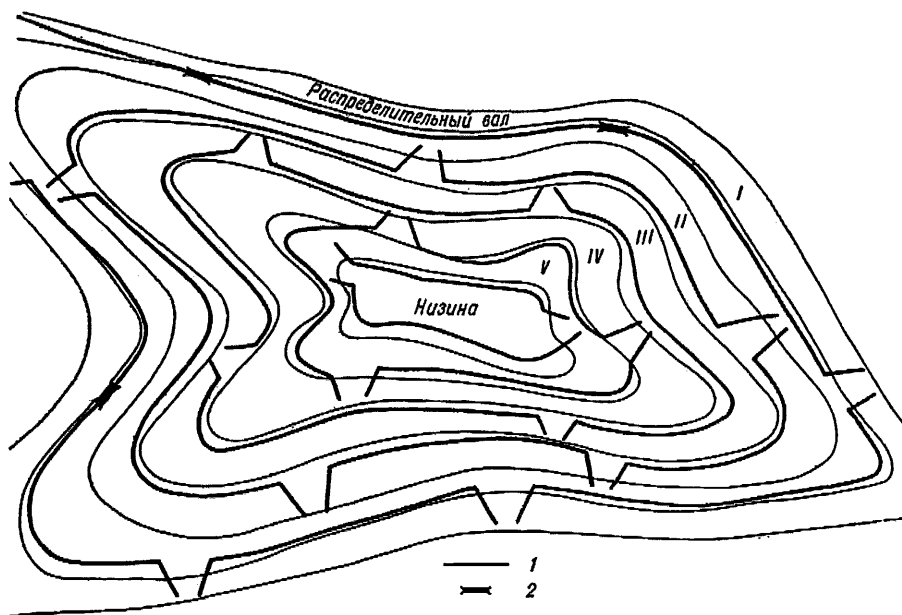
Рисунок Л.3 – Система мелкоярусных лиманов, устраиваемая у подножия больших склонов
