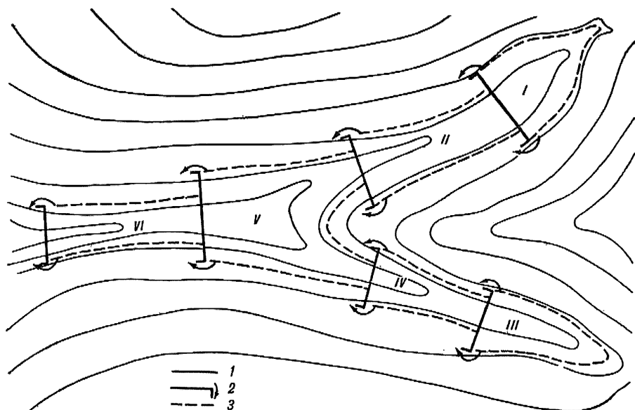
Рисунок Л.5 – Система ярусных лиманов мелкого слоя затопления, устраиваемая на потяжинах
