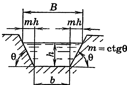
Рисунок Н.1 — Схема канала трапецидальной формы
