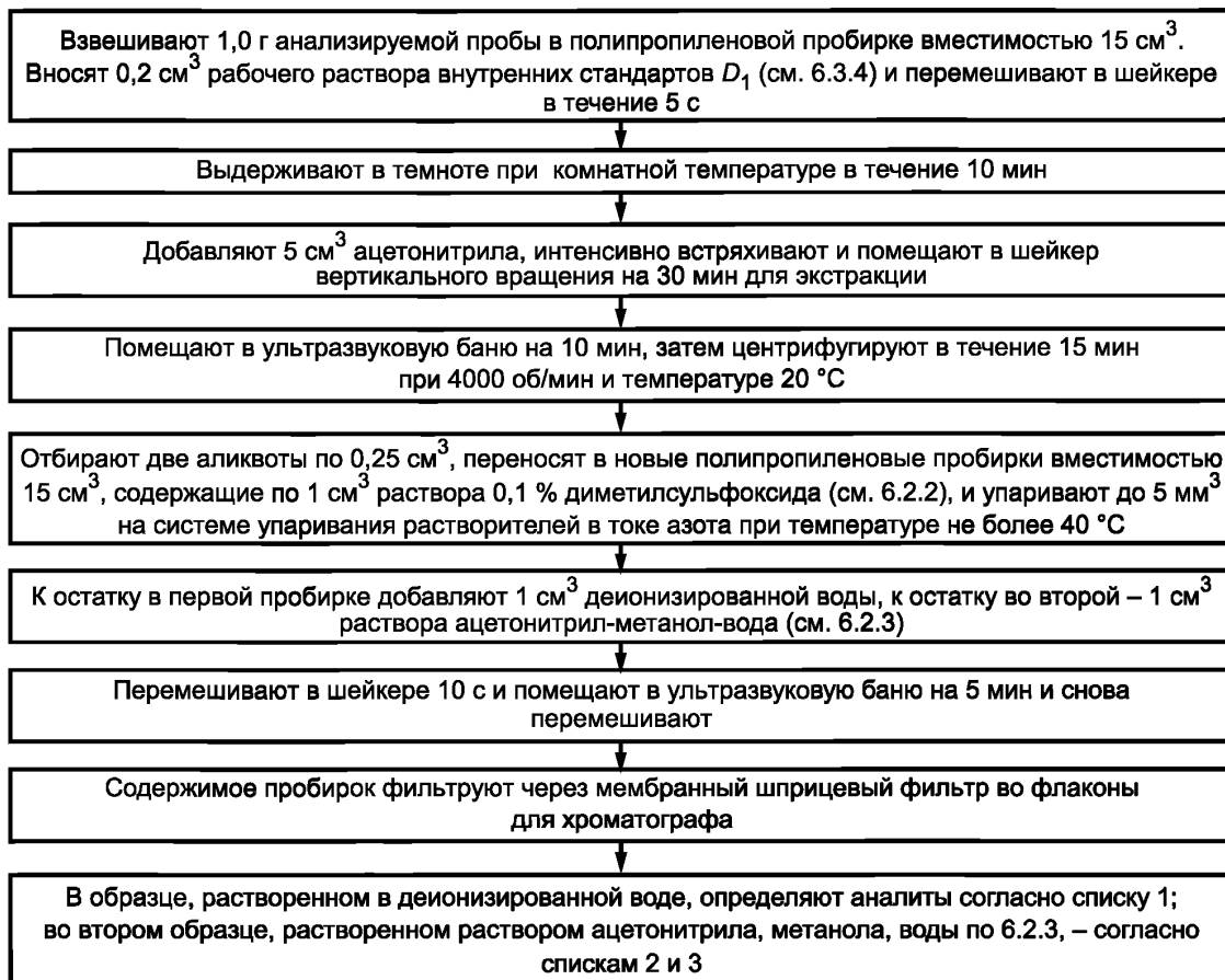
Рисунок 1 — Подготовка проб
